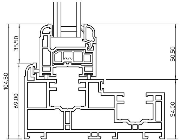
Top Jamb
